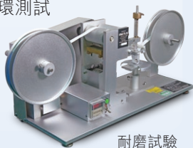
耐磨試驗
